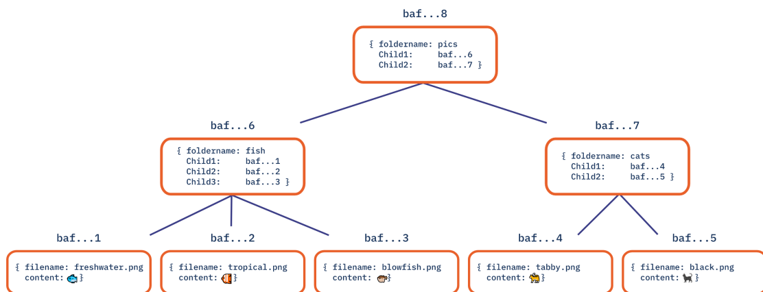
Σχήμα 2.10: Παράδειγμα Merkle DAG 10
