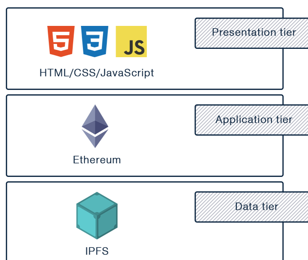
Σχήμα 3.1: Επιλεγμένη τεχνολογική στοίβα
