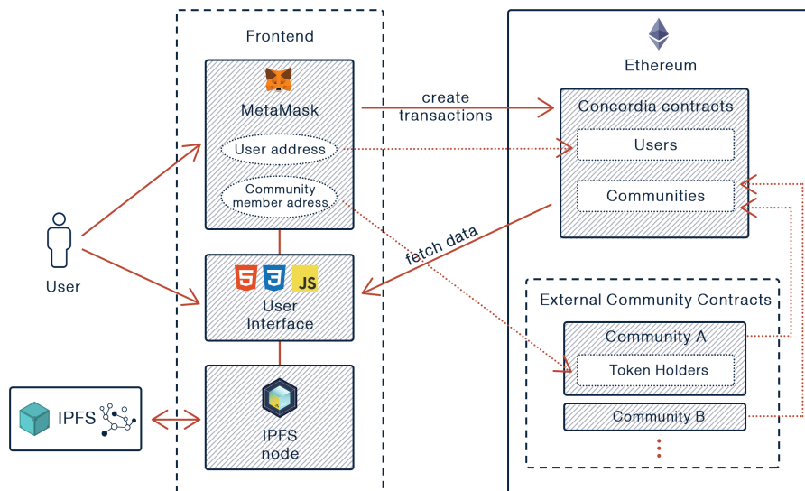
Σχήμα 3.15: Αρχιτεκτονική του συστήματος (στάδιο σχεδίασης)
